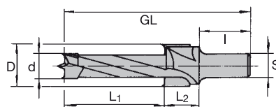
Stufenbohrer
