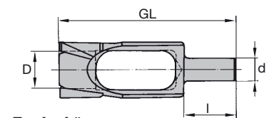
Zapfenfräser
