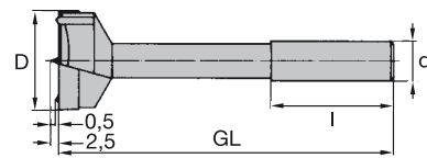
Zylinderkopfbohrer
